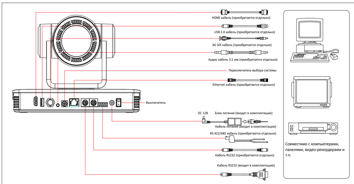
Схема интерфейсов
